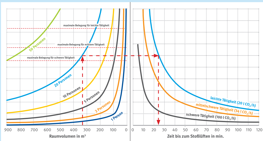
Abbildung 2: Nomogramm zur Ermittlung der Lüftungsintervalle für größere Räume
