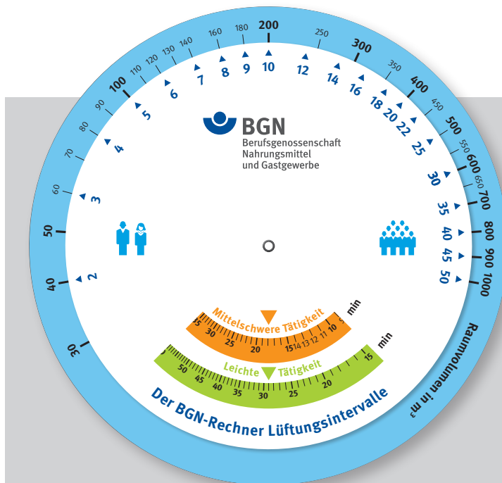
BGN-Lüftungsdrehscheibe
